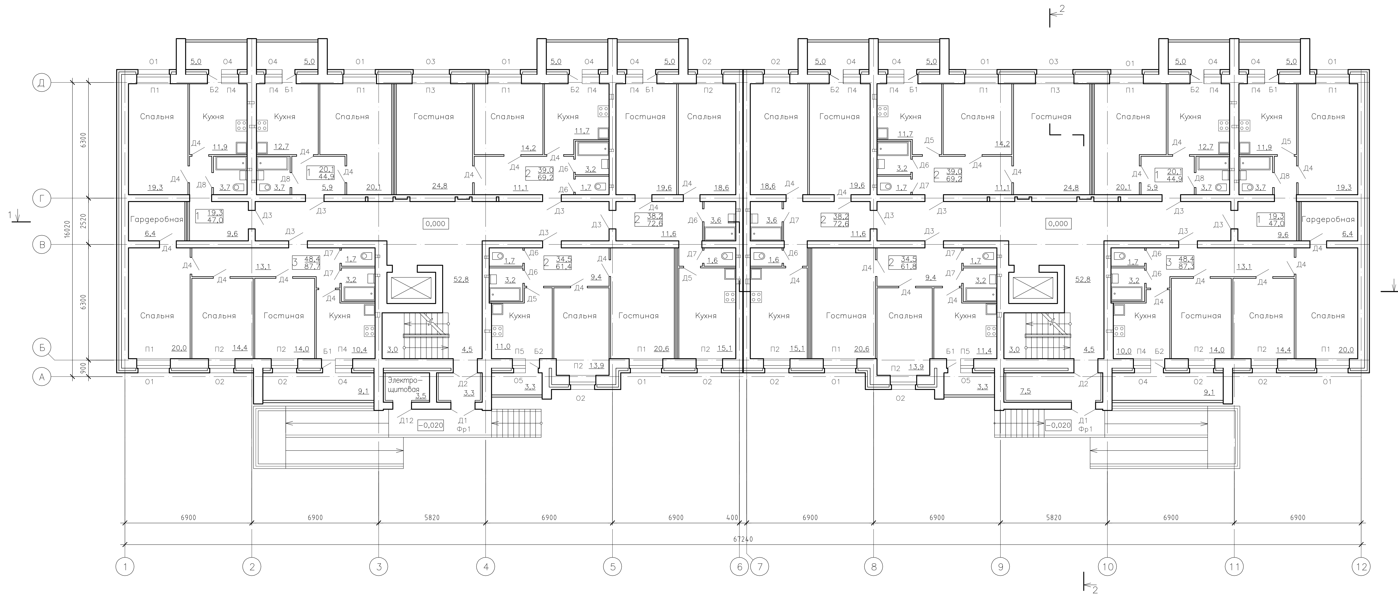
План 1 этажа
